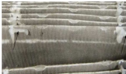
Fotografía n° 1.-Imagen de un filtro en la instalación
